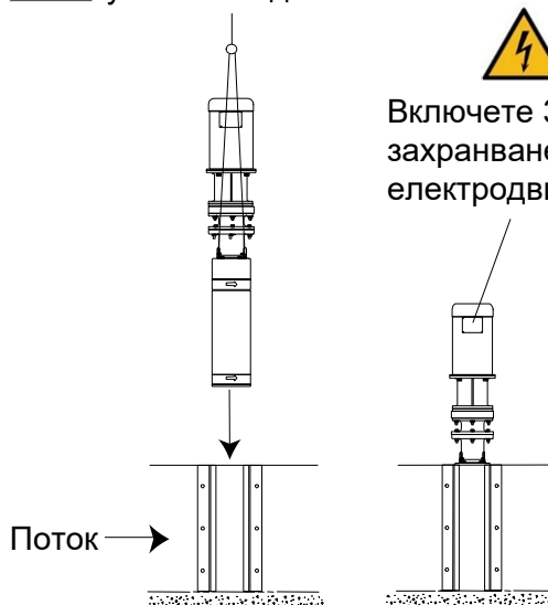
Монтаж на канал
