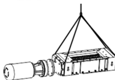
Хоризонтален монтаж
